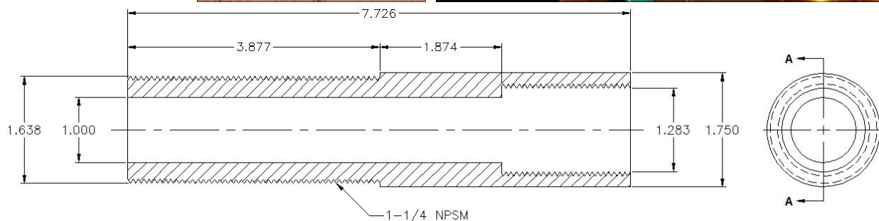
SECTION A-A
